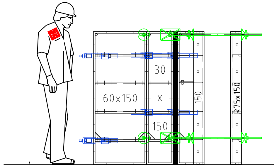
Aanzicht A-A
