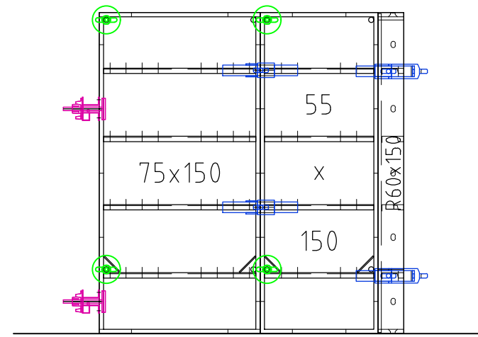
Aanzicht B-B
